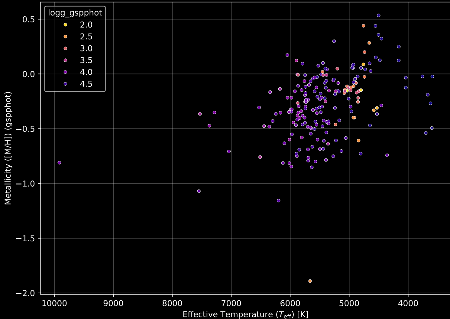
APOGEE DR17 Field: [107-46_MGA] Stellar Population Parameters (n= 200)
